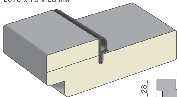
Коробка прямая, МДФ, с уплотнителем 2070 x 70 x 28 мм
