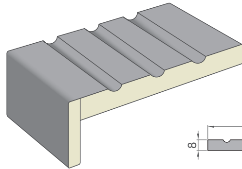
Наличник фигурный, телескоп 2150 x 75 x 26 мм
