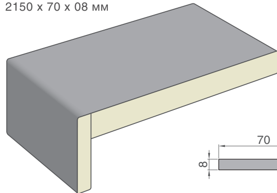
Наличник прямой, телескоп 2150 x 70 x 08 мм
