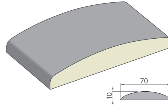
Наличник полукруглый 2150 x 70 x 10 мм
