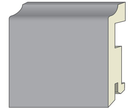
Плинтус напольный П-22, МДФ, с кабель каналом 2070 x 81 x 16 мм
