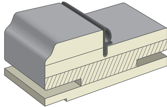
Наличник каннелюр, телескоп 2150 x 70 x 08 мм
